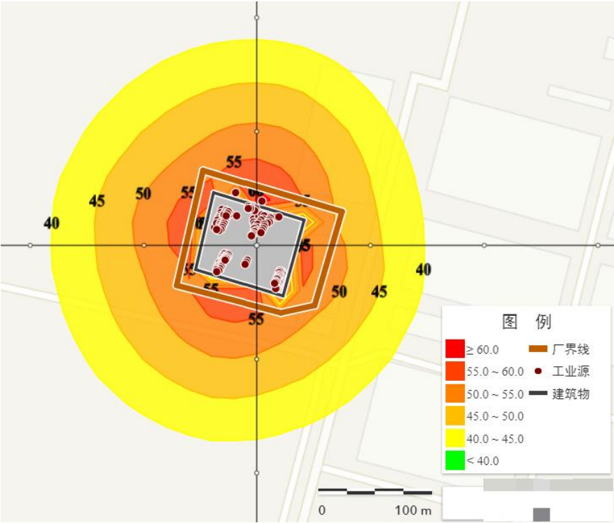
图 4-3 项目预测等声级线图
