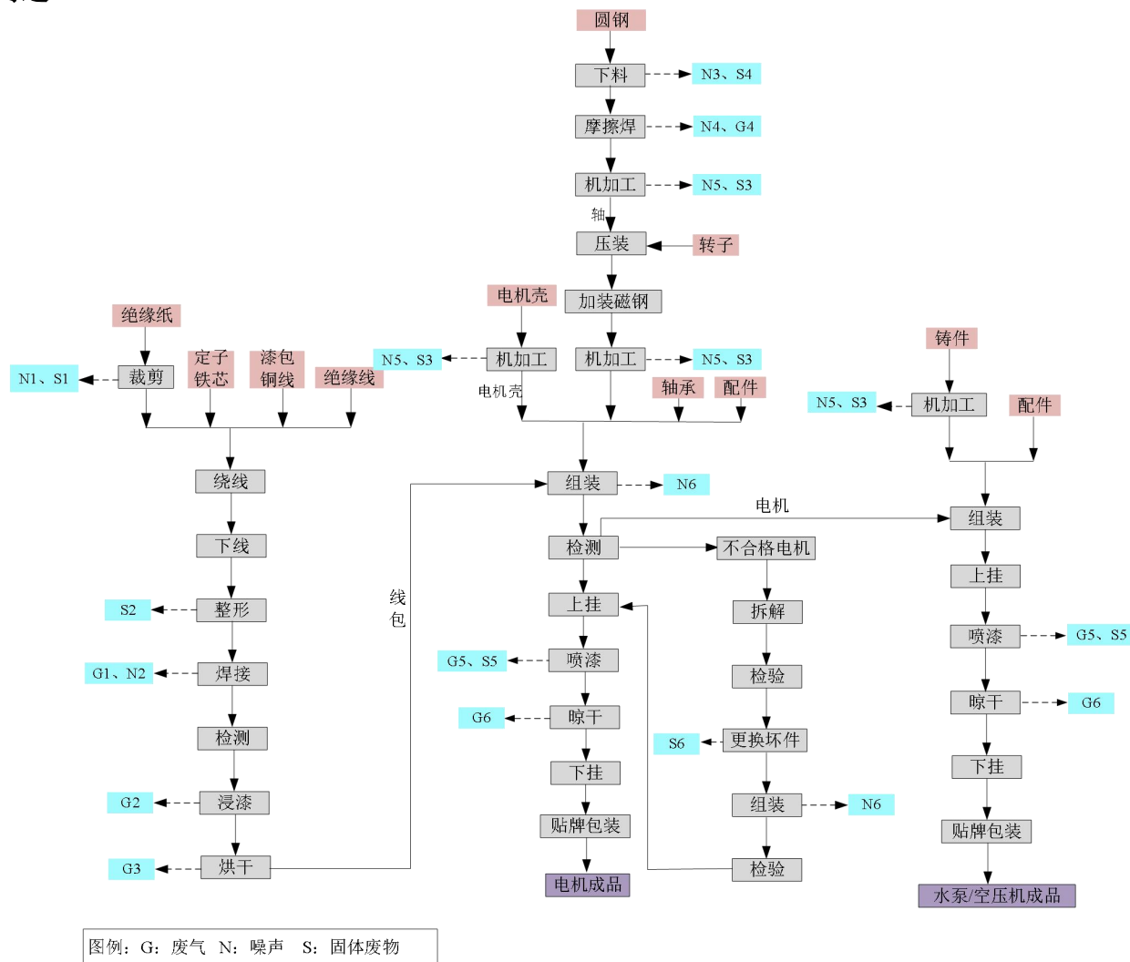
图 2-2 本项目生产工艺和产排污节点图
