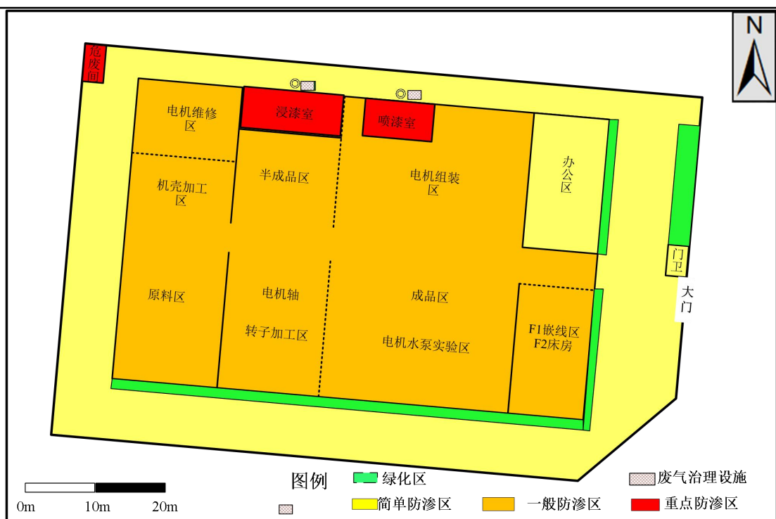
图 4-4 厂区分区防渗图
