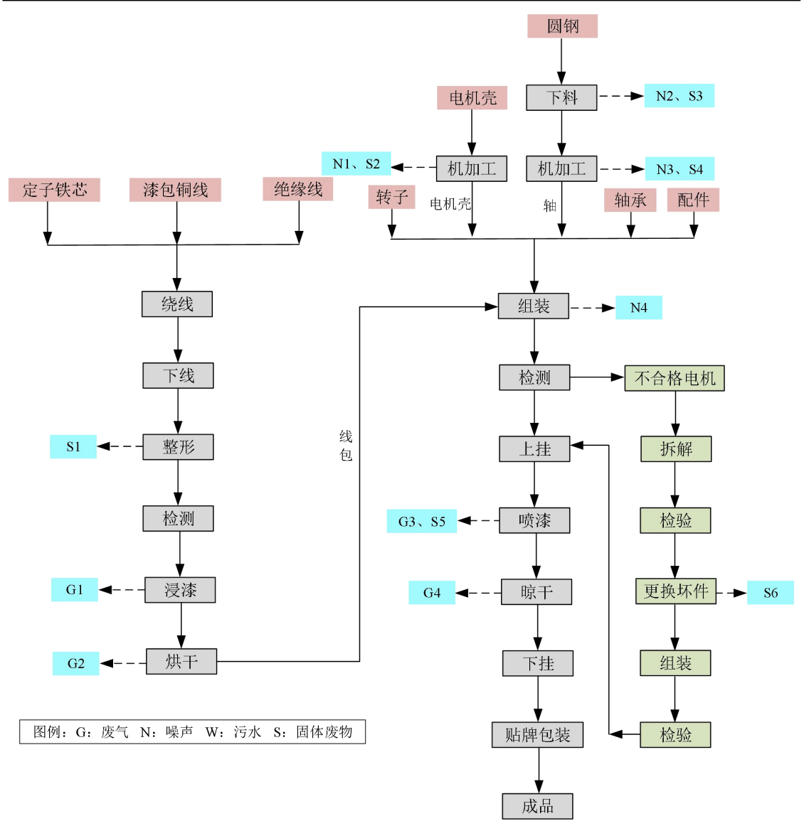
图 2-3 生产工艺及排污图
