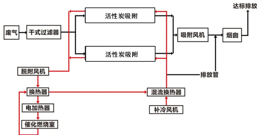
图 4-2 吸附脱附+催化燃烧废气治理设施工艺图
