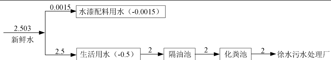
图 2-1 本项目水平衡图 (m³/d)
