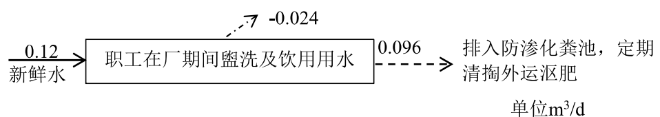
图2-3现有项目水平衡图
