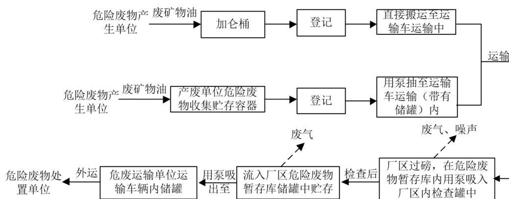
图2-4现有项目工艺流程及排污节点图
