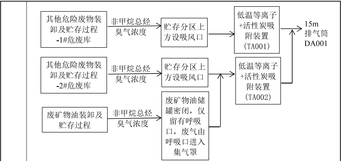
图 4-1 废气治理设施配置图
