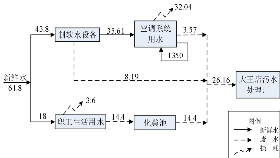
图 5 扩建项目完成后全厂春、秋季水平衡图（单位：m³/d）
