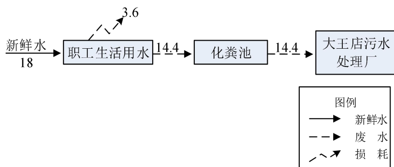
图 4 扩建项目完成后全厂冬季水平衡图 (单位: \text{m}^3/\text{d} )
