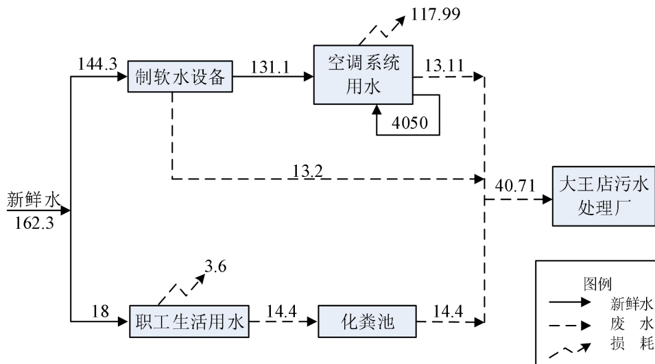
图 5 扩建项目完成后全厂春、秋季水平衡图（单位：m³/d）
