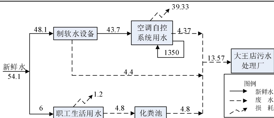
图 2 项目夏季水平衡图 (单位: \text{m}^3/\text{d} )
